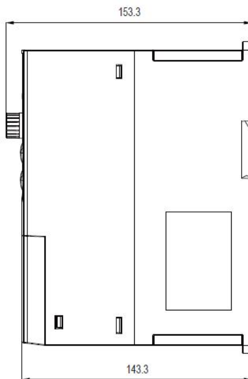
HC10 标准版 3.7kW—5.5kW 结构示意图及尺寸
