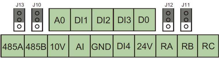
HC10M 版 0.75K-1.5KW 控制回路端子布置图：
