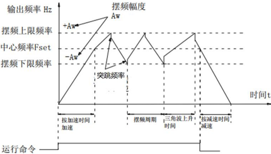
摆频工作示意图
