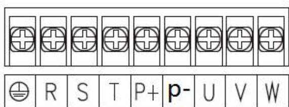
3.7kW-11kW 主回路端子示意图
