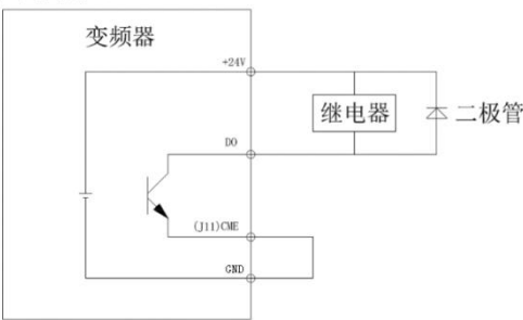
数字输出端子接线示意图
