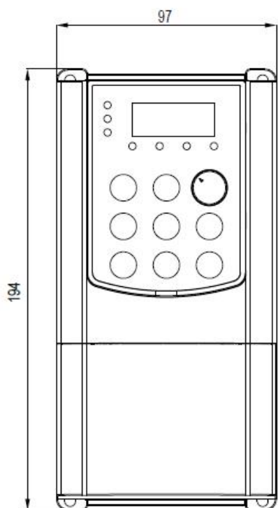
HC10 标准版 3.7kW—5.5kW 结构示意图及尺寸
