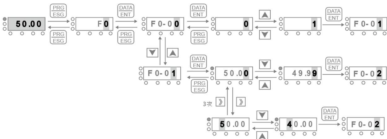
修改参数示意图
