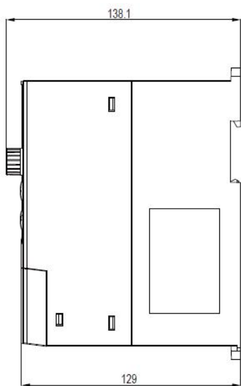
HC10 标准版 0.75KW-2.2kW 结构示意图及尺寸
