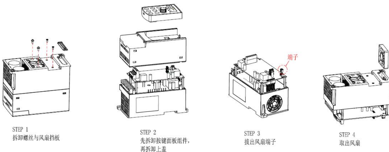
0.75KW~5.5KW 机器风扇维护示意图
