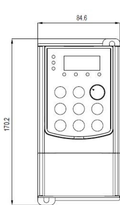
HC10 标准版 0.75KW-2.2kW 结构示意图及尺寸
