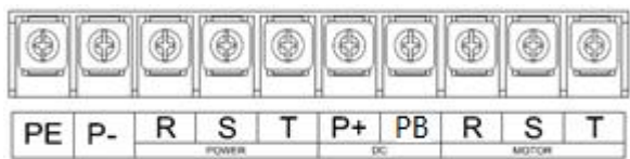
15kW-22kW 主回路端子示意图
