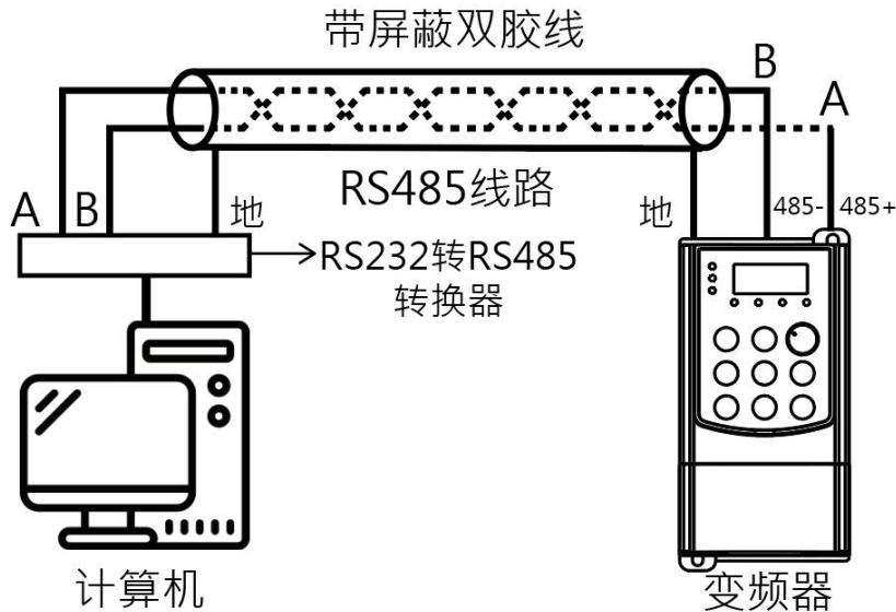
RS485 单机应用时的物理接线图
