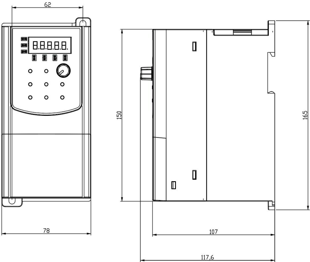
HC10M 0.75KW-1.5kW 结构示意图及尺寸
