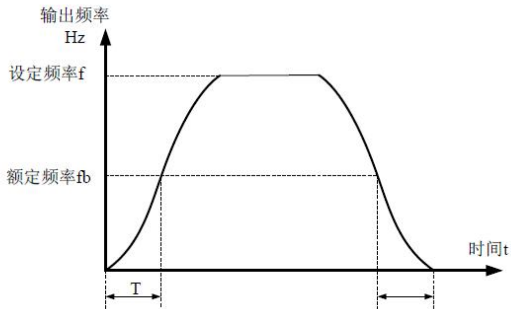
S曲线加减速B示意图
