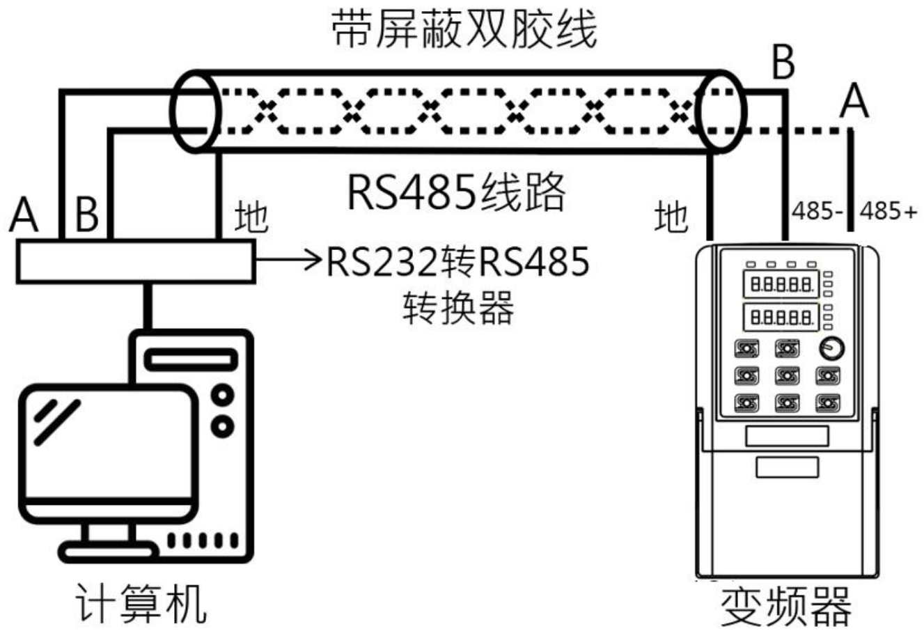
RS485 单机应用时的物理接线图
