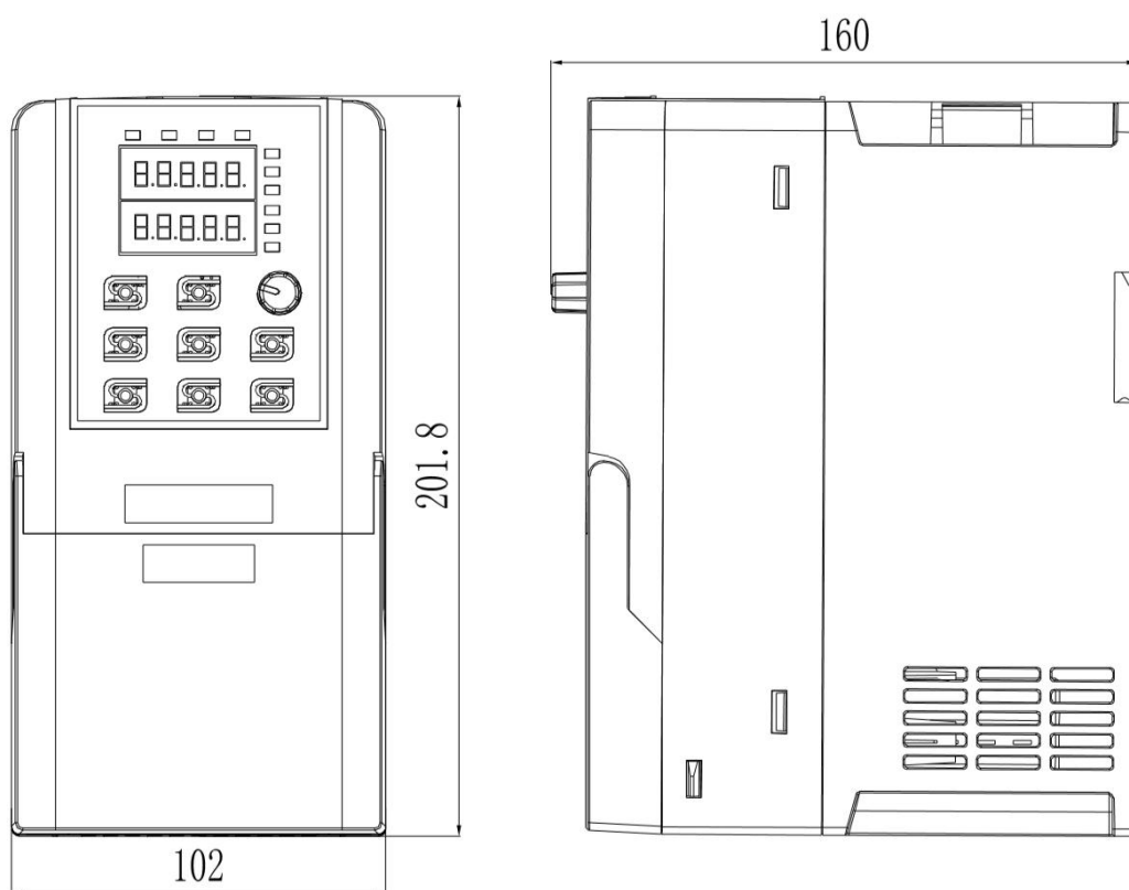
3.7kW—5.5kW 结构示意图及尺寸
