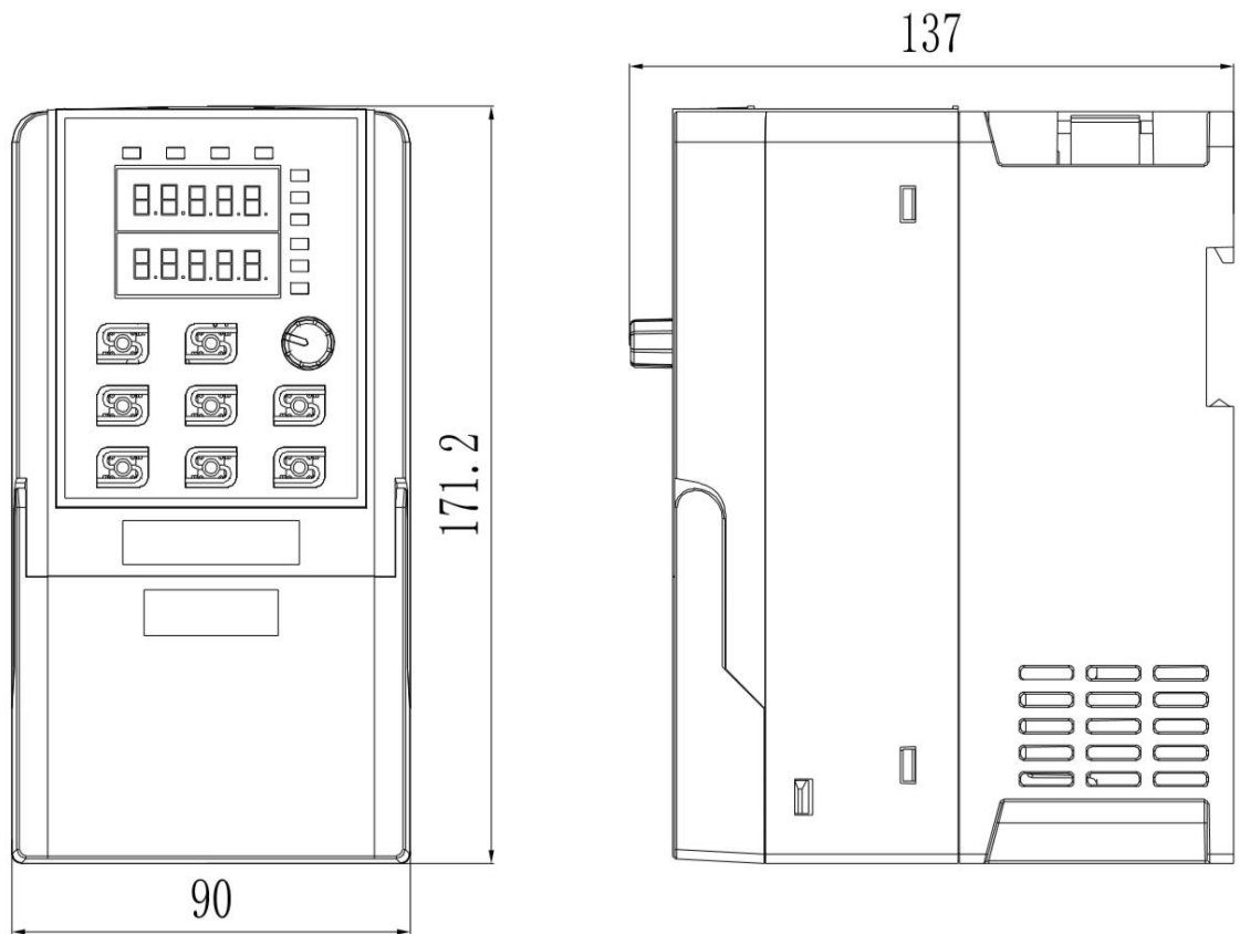
0.75kW—2.2kW 结构示意图及尺寸
