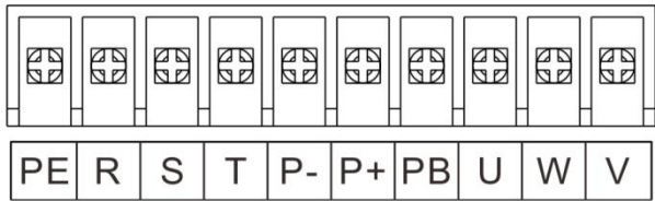
3.7kW-22kW 主回路端子示意图
