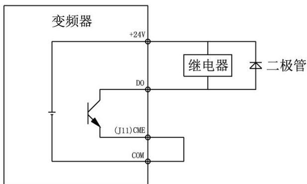
数字输出端子接线图
