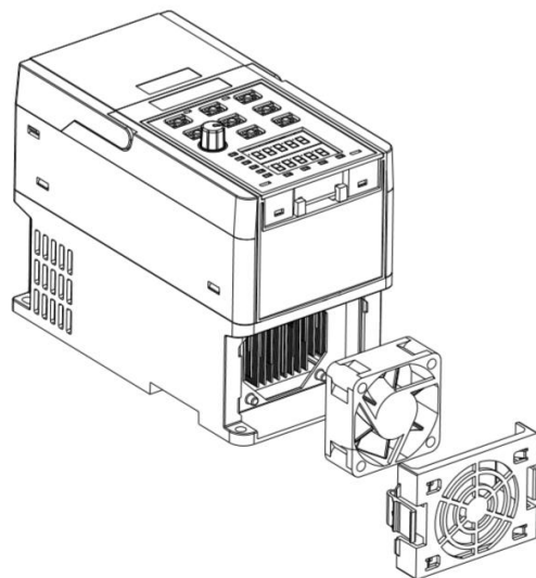
STEP 2 取出风扇并拔出风扇电源端子
