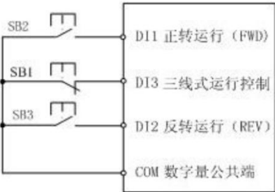
三线式模式 1
