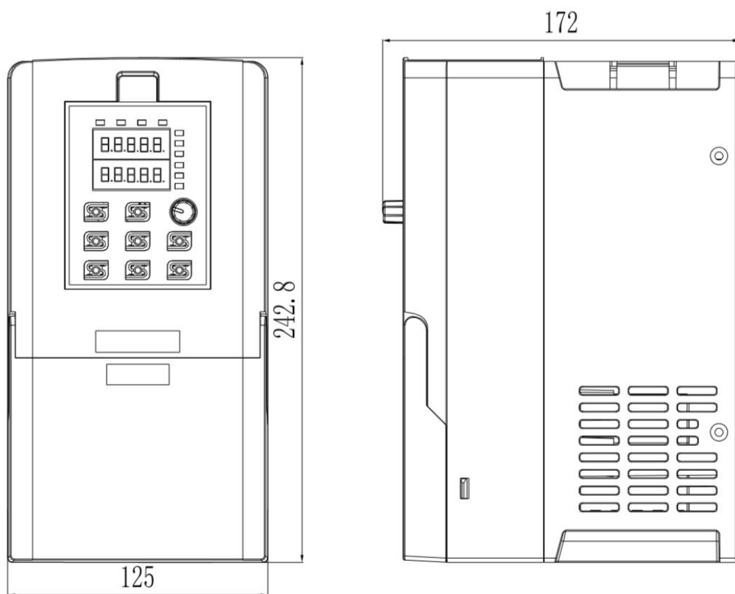
7.5kW—11kW 结构示意图及尺寸
