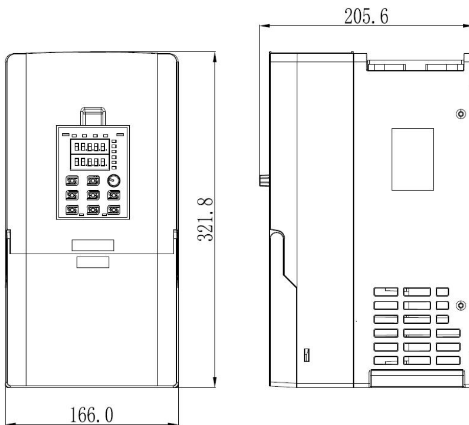
15kW—22kW 结构示意图及尺寸
