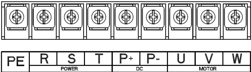
30kW-37kW 主回路端子示意图
