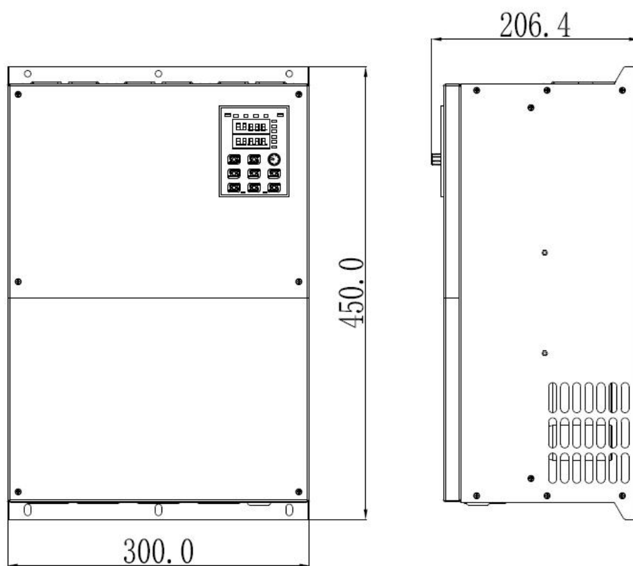
30kW—37kW 结构示意图及尺寸
