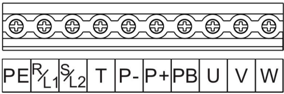
0.75kW-2.2kW 主回路端子示意图
