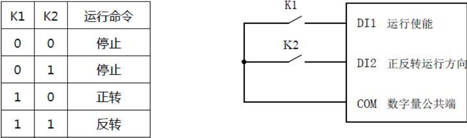
两线式模式 2
