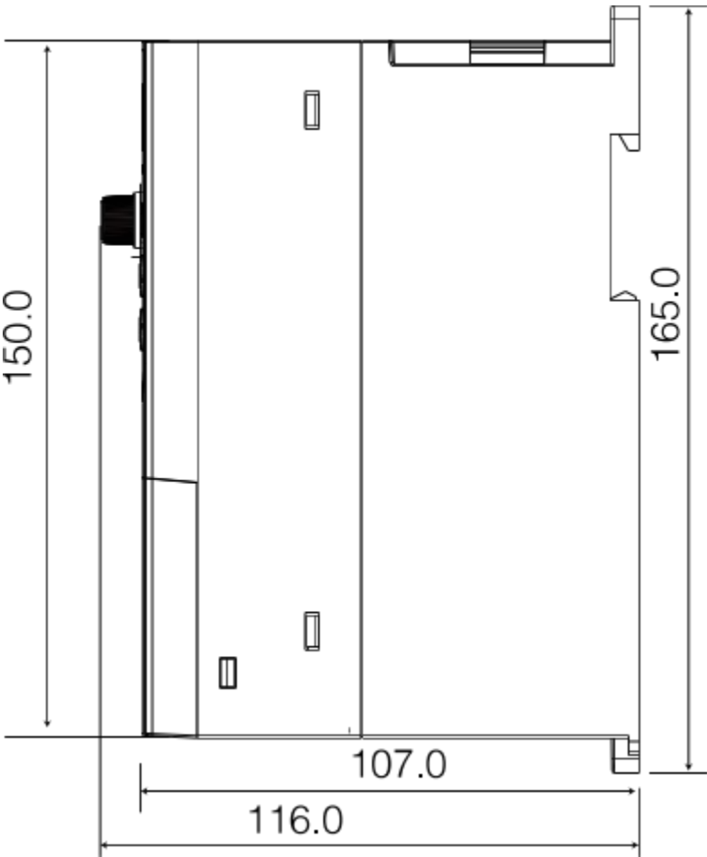
0.75kW—2.2kW 结构示意图及尺寸
