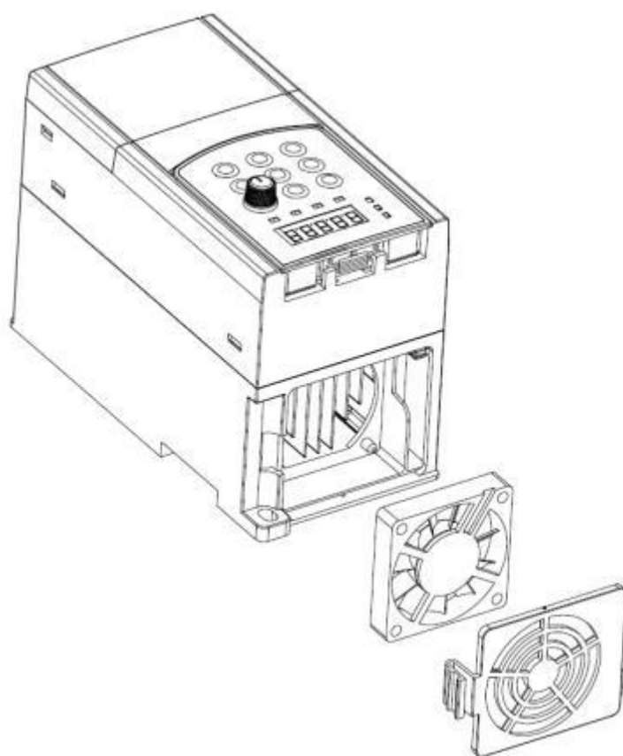
0.75kW~2.2kW 机器风扇维护示意图
