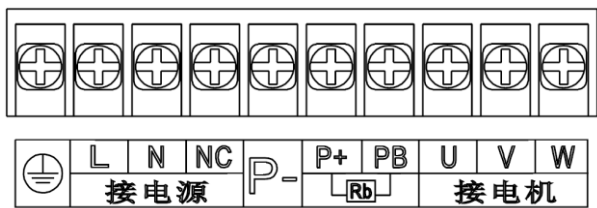
0.75kW-2.2kW 单相主回路端子示意图
