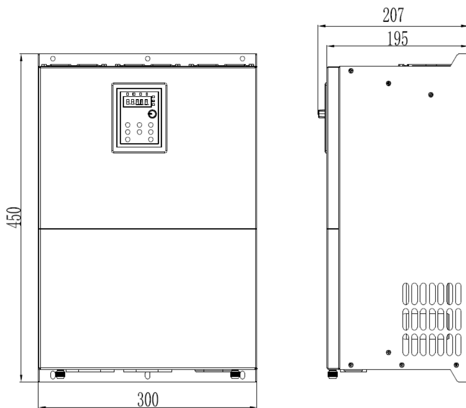
30kW—37kW 结构示意图及尺寸
