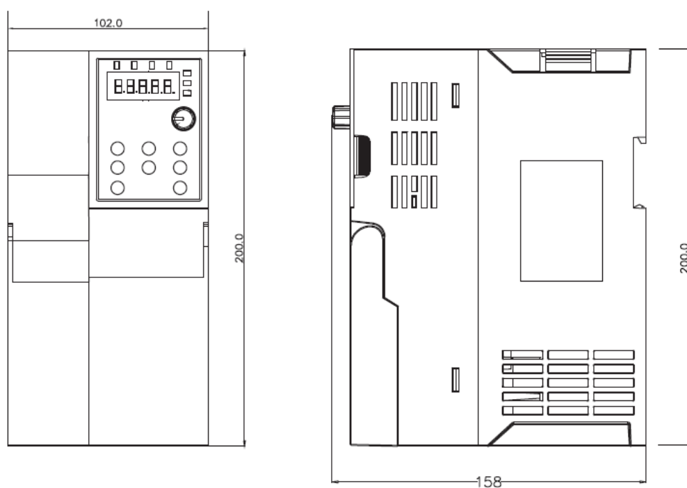
3.7kW—5.5kW 结构示意图及尺寸
