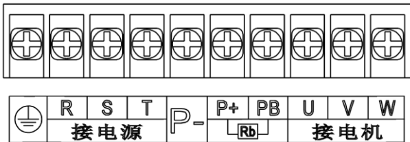
0.75kW-5.5kW 三相主回路端子示意图
