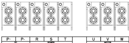
45kW-55kW 三相主回路端子示意图
