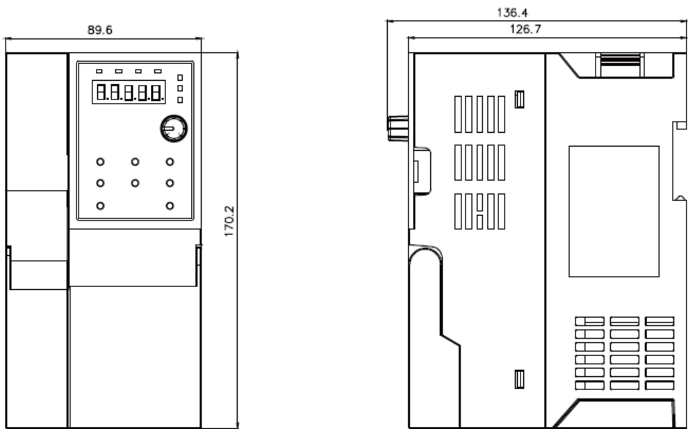
0.75kW—2.2kW 结构示意图及尺寸
