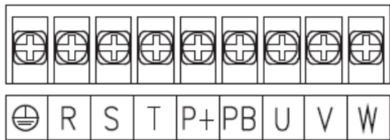
7.5kW-11kW 三相主回路端子示意图
