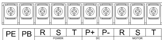
30kW-37kW 三相主回路端子示意图
