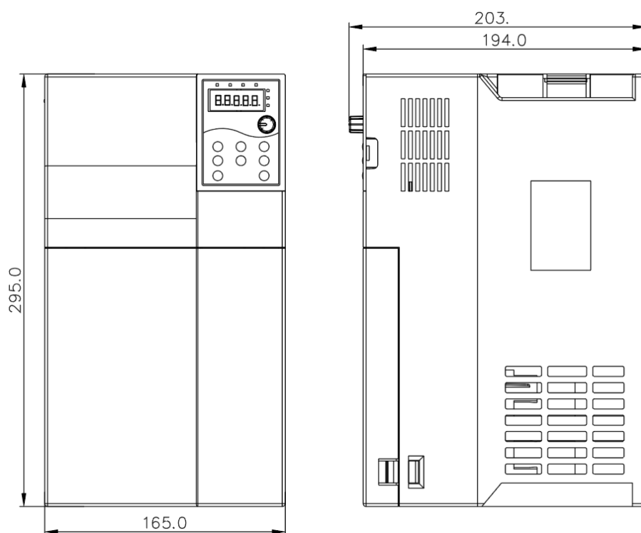
15kW—22kW 结构示意图及尺寸
