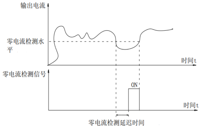
零电流检测示意图
