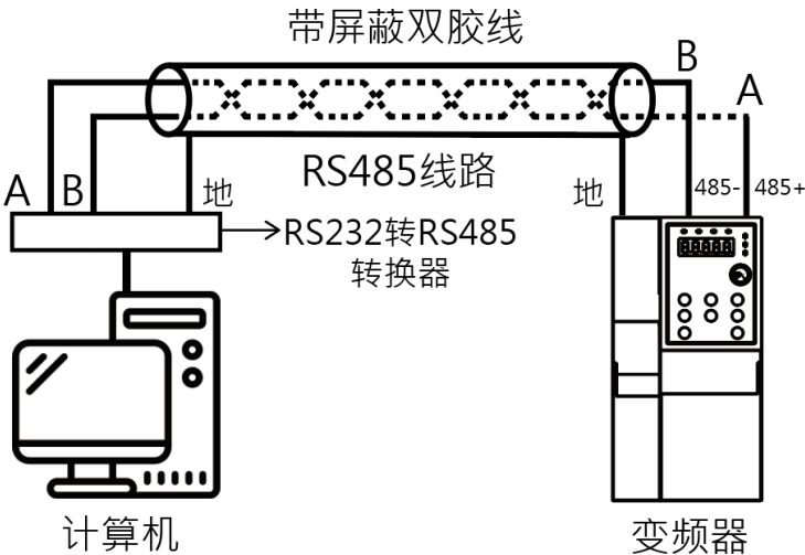
RS485 单机应用时的物理接线图
