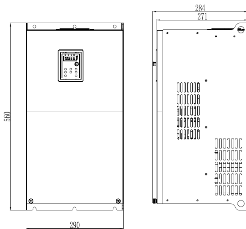
45kW—55kW 结构示意图及尺寸
