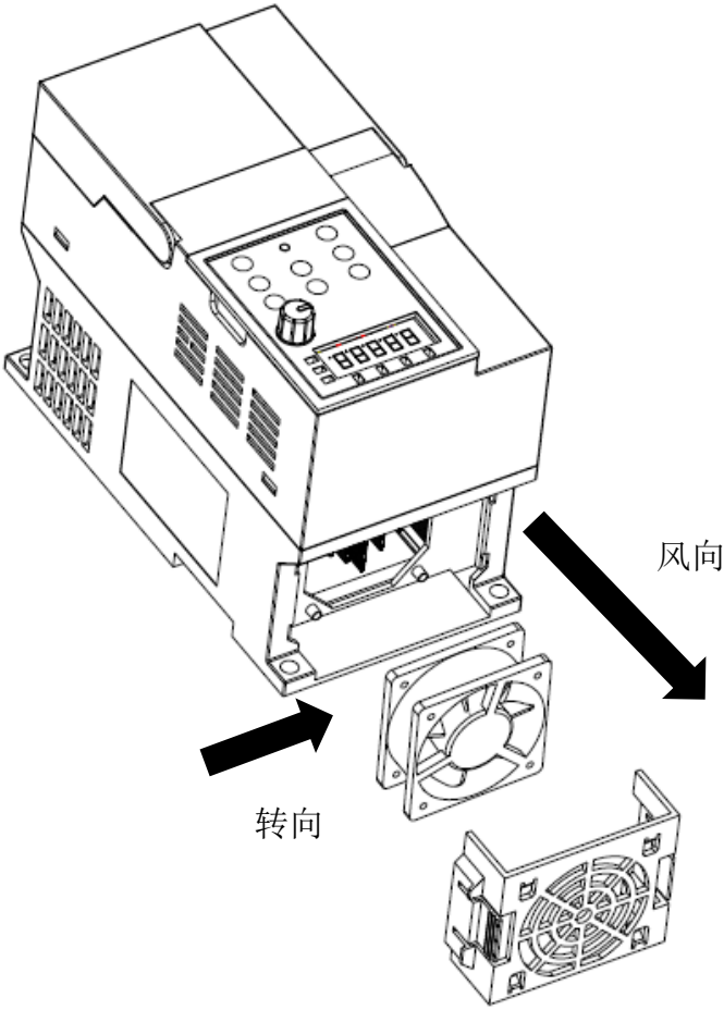
机器风扇维护示意图
