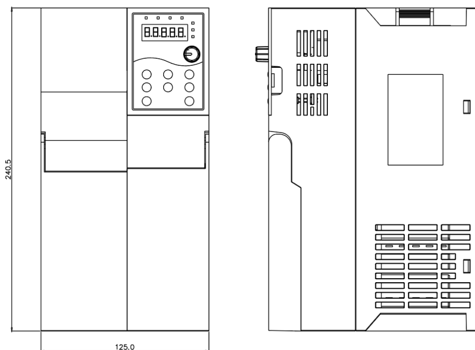
7.5kW—11kW 结构示意图及尺寸
