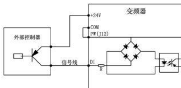
使用内部 24V 电源的 PNP 漏型连接方式
