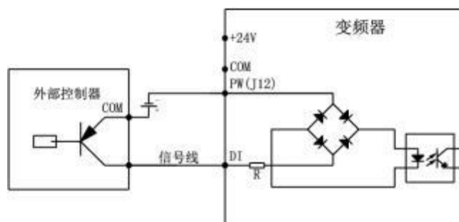
使用外部电源的 PNP 漏型连接方式 (注意 J12 去除 PW 与 +24V 之间的跳线)
