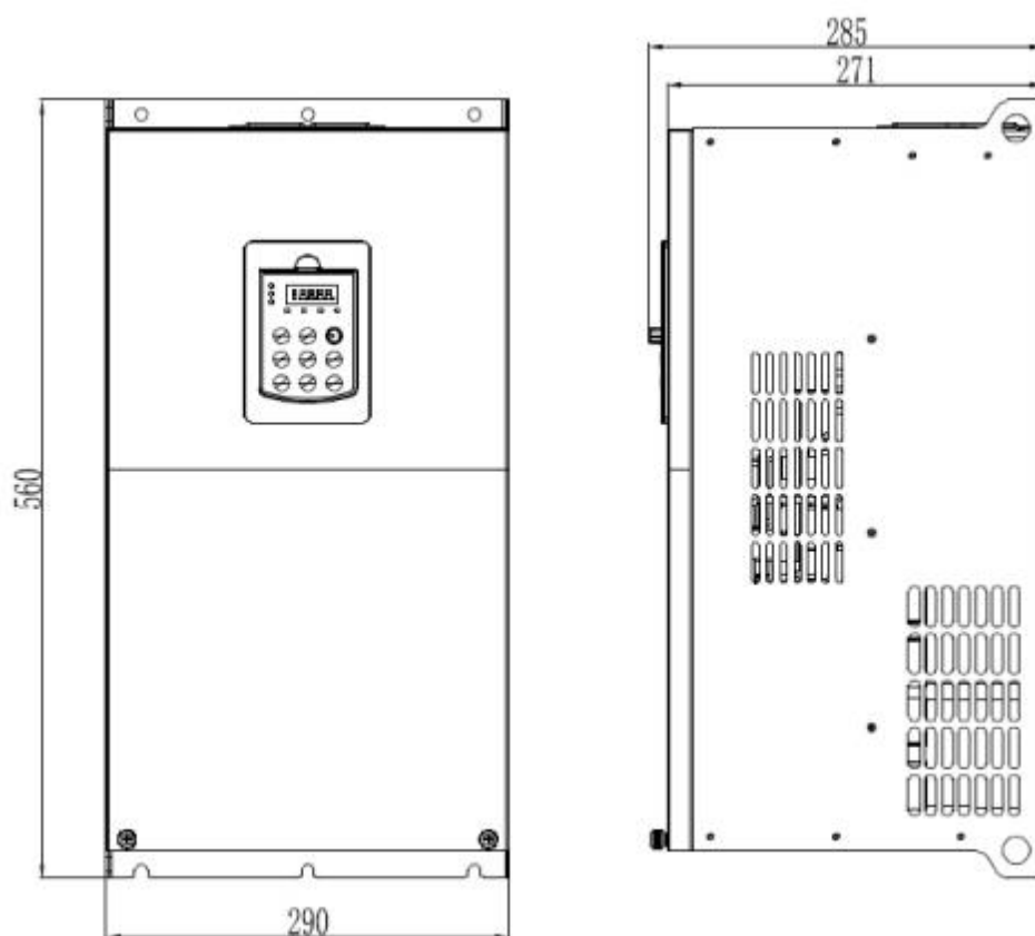
45kW—55kW 结构示意图及尺寸
