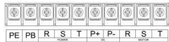
30kW-37kW 主回路端子示意图
