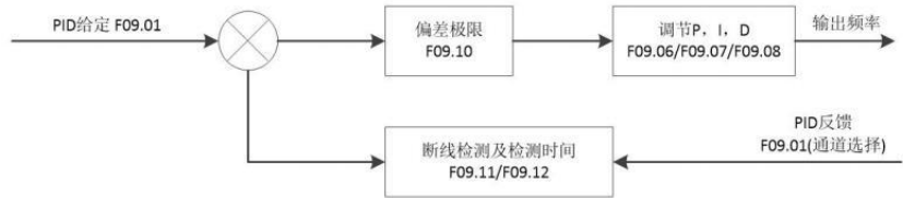
图 5-11 PID 控制原理
