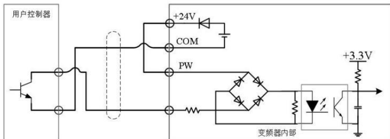
图 2-6 NPN 型灌电流接线方式
