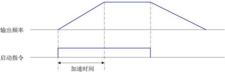
图 5-13 直接启动时序图
