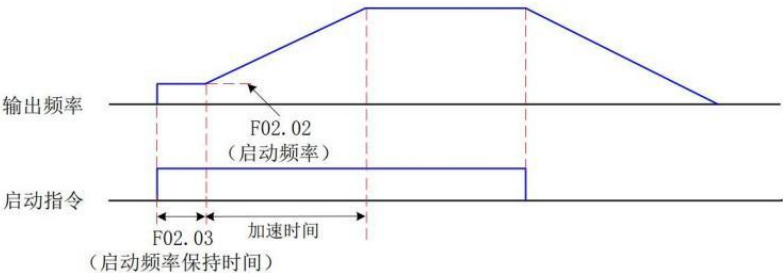
图 5-14 带启动频率的启动时序图
