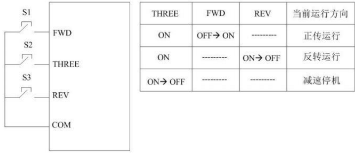
图 5-4 三线式控制 2
