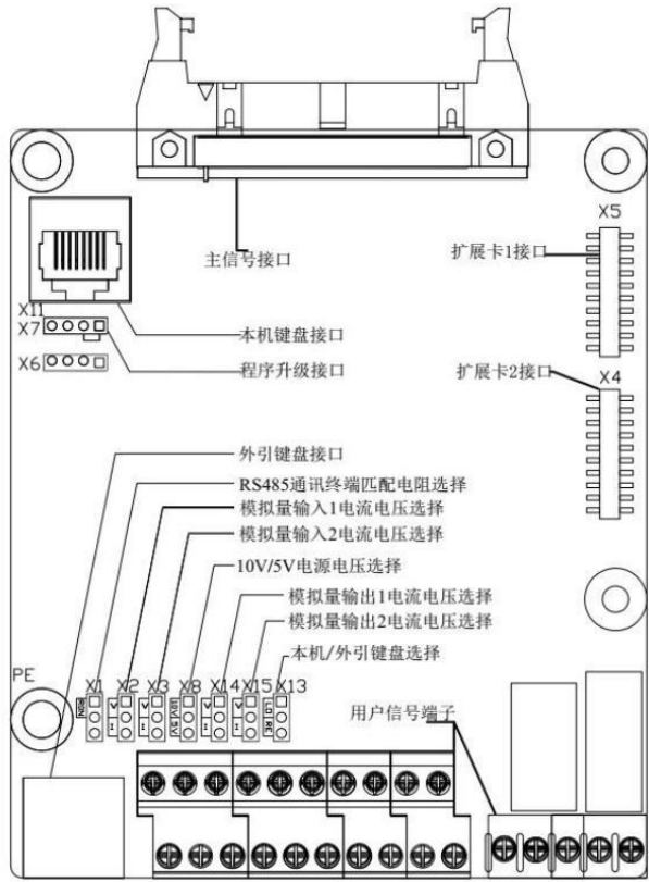
图 2-3 控制板示意图
