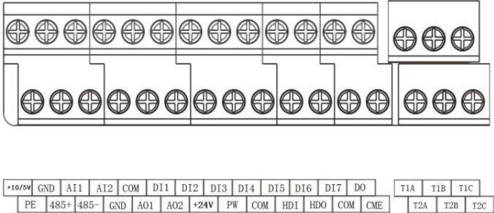
图 2-4 控制板端子示意图
