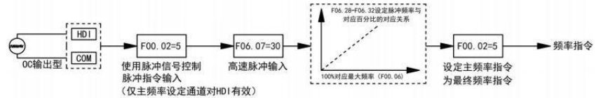
图 5-9 脉冲给定输入主频率参数设置
