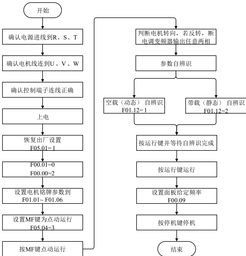
图 3-2 首次上电流程图
