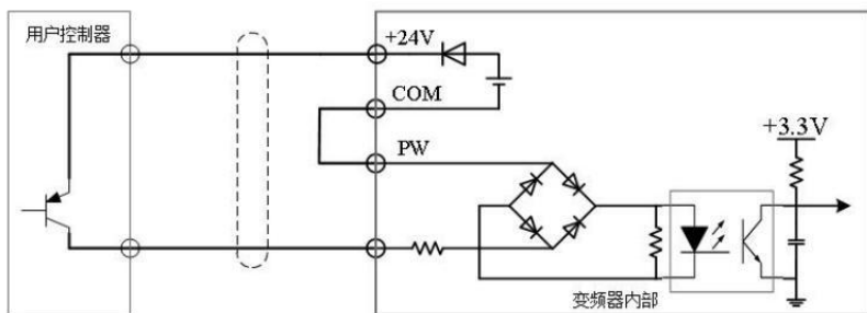
图 2-7 PNP 型拉电流接线方式
