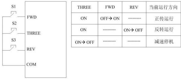
图 5-3 三线式控制 1
