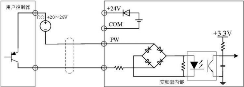
图 2-9 PNP 型拉电流接线方式
