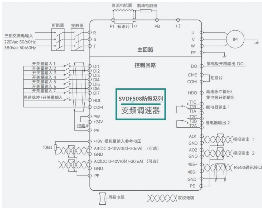
图 2-2 标准接线图
