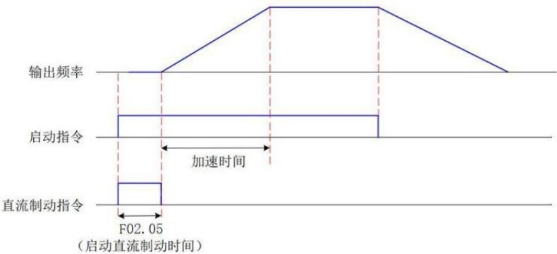
图 5-15 带直流制动的启动时序图
