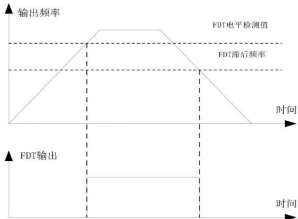
图 5-17 输出频率与 FDT 输出关系图
