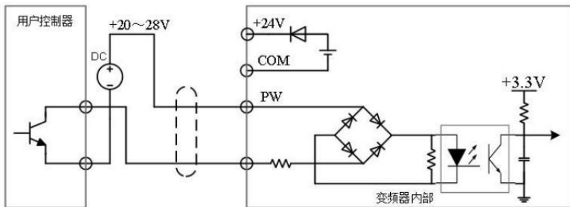
图 2-8 NPN 型灌电流接线方式
