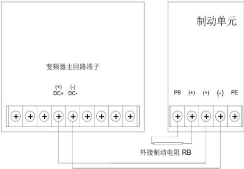
外置制动单元接线
