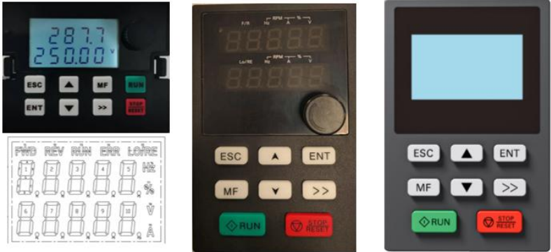
图 5-3 选配 LCD 键盘
