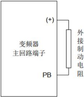
内置制动单元接线
