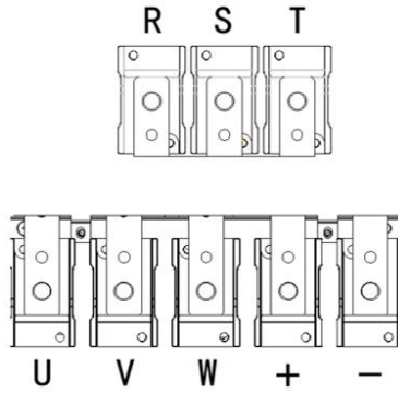
图 4-17 三相 380V 132~160kW 主回路端子 (单位: mm)
