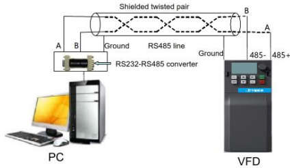
图 10-1 RS485 单机应用时的物理接线
