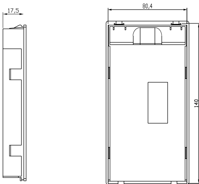
图 B 22KW 以上外引键盘支架 (键盘托) 外形尺寸图 (单位 mm)
