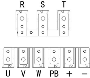
图 4-16 三相 380V 75~110kW 主回路端子 (单位: mm)
