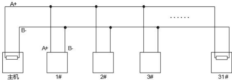
图 10-2 菊花接法现场接线
