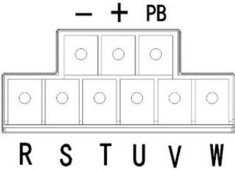
图 4-15 三相 380V 18~37kW 主回路端子（单位：mm）
