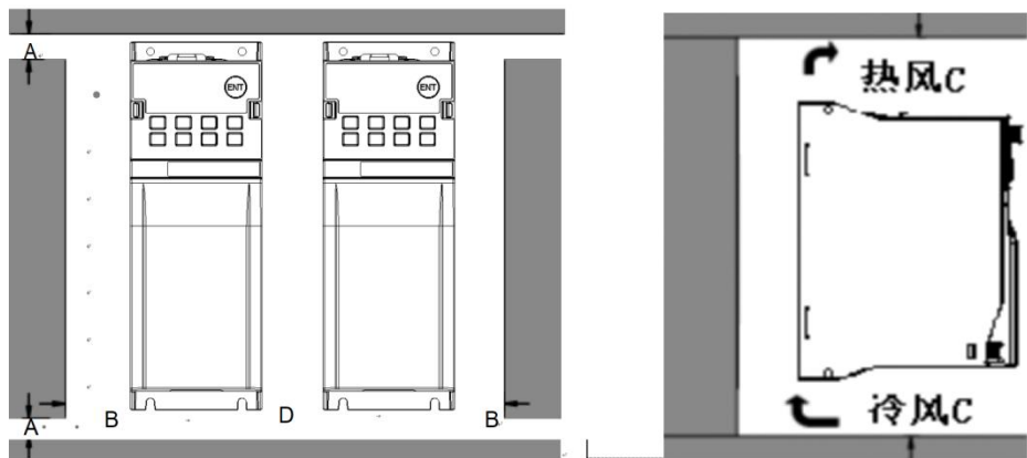
图 4 并行安装
