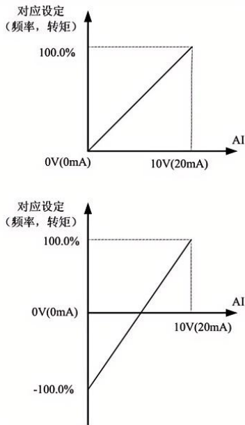
图 F07-6 模拟给定与设定量的对应关系
