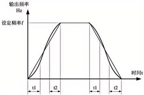
图 F01-1 曲线加减速 A 示意图
