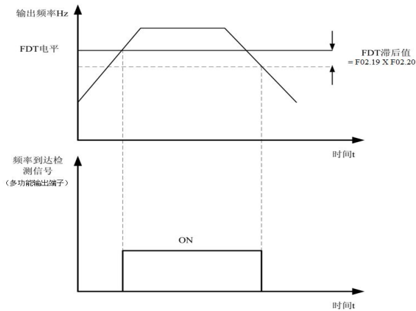
图 F01-6 FDT 电平示意图
