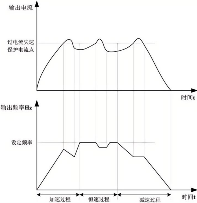
图 F12-1 过流失速保护示意图
