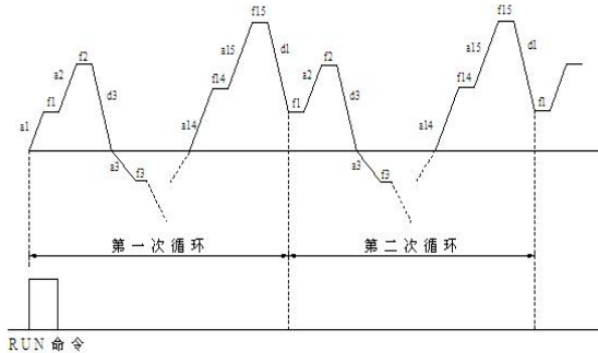
图 F10-3 PLC 一直循环示意图
