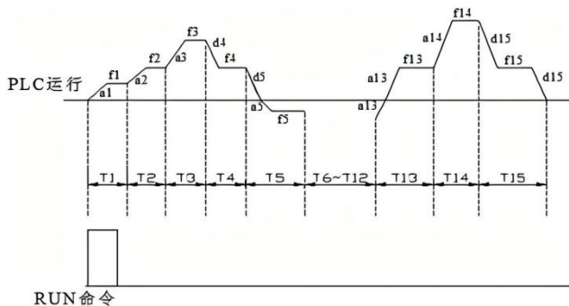
图 F10-1 PLC 单次循环后停机示意图
