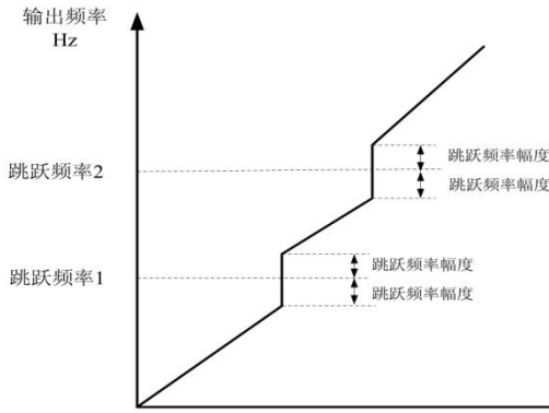
图 F01-8 加减速过程中跳跃频率有效示意图
