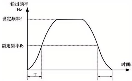
图 F01-2 曲线加减速 B 示意图
