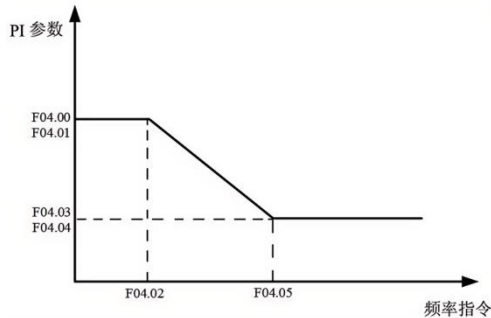
图 F04-1 PI 参数示意图
