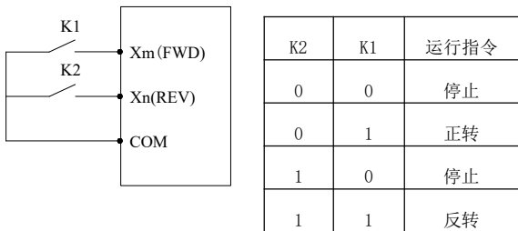
图 F07-2 二线式控制模式 1 示意图
