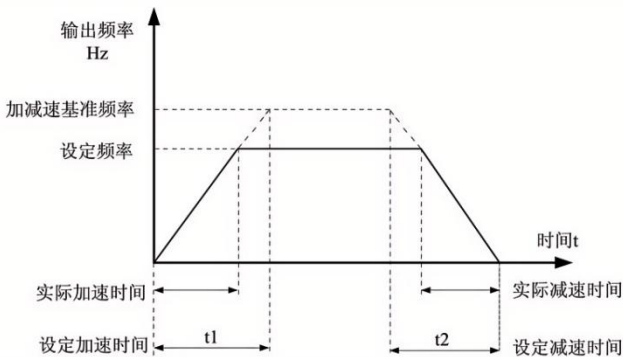
图 F00-1 加速时间和减速时间示意图
