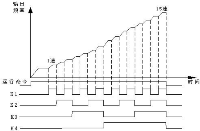
图 F07-1 多段速运行示意图
