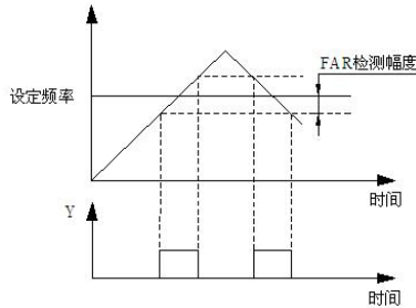
图 F01-7 频率到达检出幅值示意图
