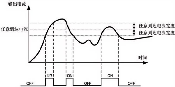
图 F01-12 任意到达频率检测示意图
