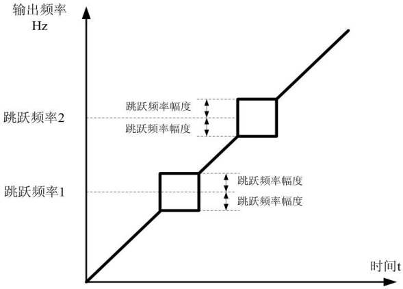
图 F01-4 跳跃频率示意图
