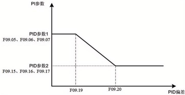
图 F09-1 PID 参数切换
