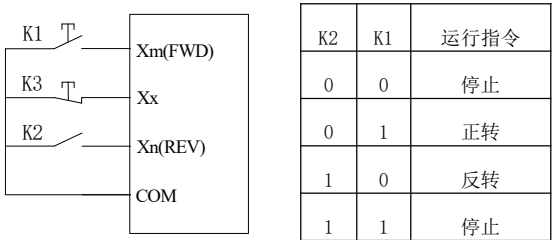
图 F07-5 三线式控制模式 2 示意图
