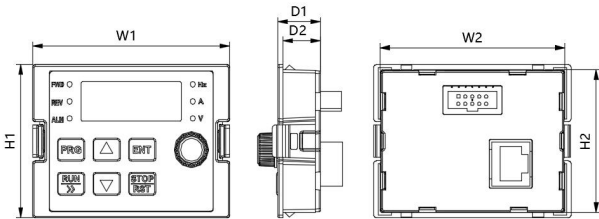
键盘安装尺寸:
