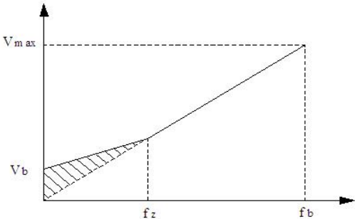
Vb-手动转矩提升量 图 F06-1 转矩提升示意图
