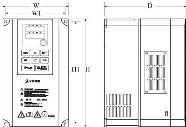
图2-3机箱外形B
