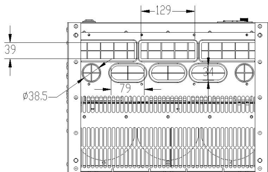
图 3-6 SVD110-185G-4~280G-4 过线圈外形尺寸图 (单位 mm)
