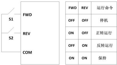
图 6-1 两线式 1
