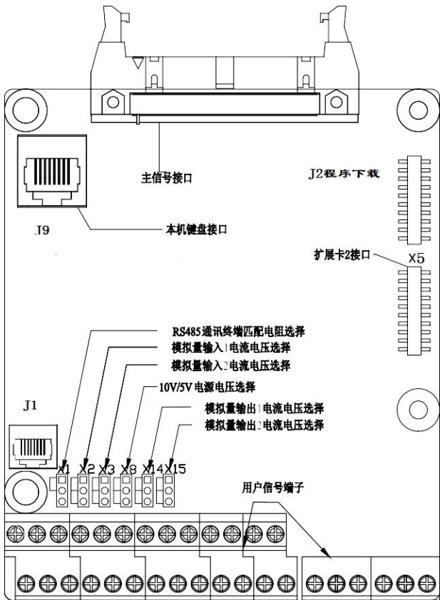
图 3-13 控制板示意图
