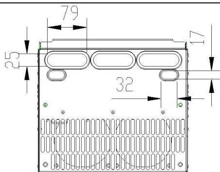
图 3-4 SVD110-055G-4~SVD110-110-4 过线圈外形尺寸图 (单位 mm)
