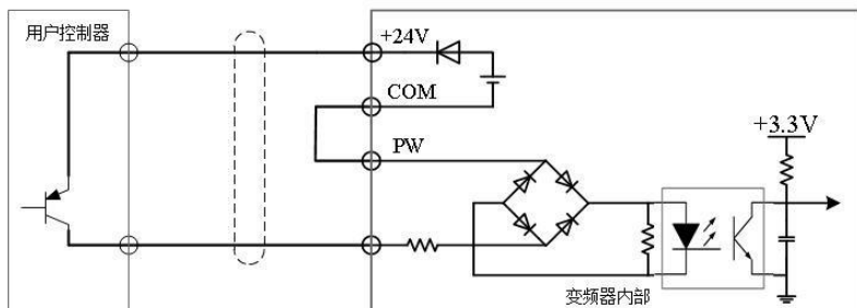
图 3-17 PNP 型拉电流接线方式
