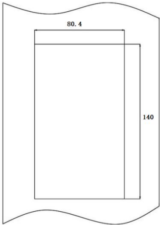
图 2-7 操作面板支架（键盘托）外引开孔尺寸图
