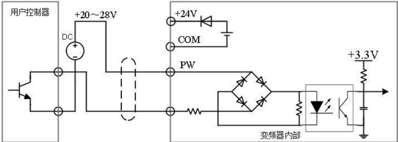
图 3-18 NPN 型灌电流接线方式注：务必去除+24V 与 PW 端子间短路片
