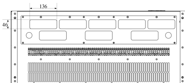
图 3-7 SVD110-315G-4~400G-4 过线圈外形尺寸图（单位 mm）
