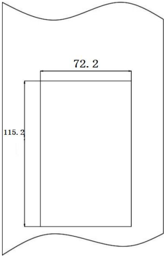
图 2-6 操作面板（键盘）本体外引开孔尺寸图 注：使用面板支架时钣金厚度不能超过 2 毫米
