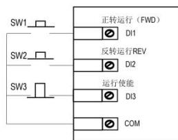
图 6-3 三线式1
