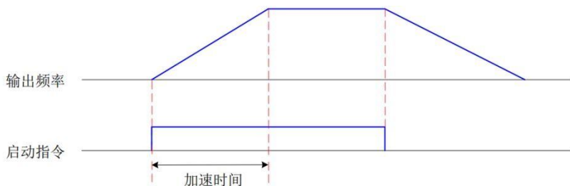
图 6-13 直接启动时序图
