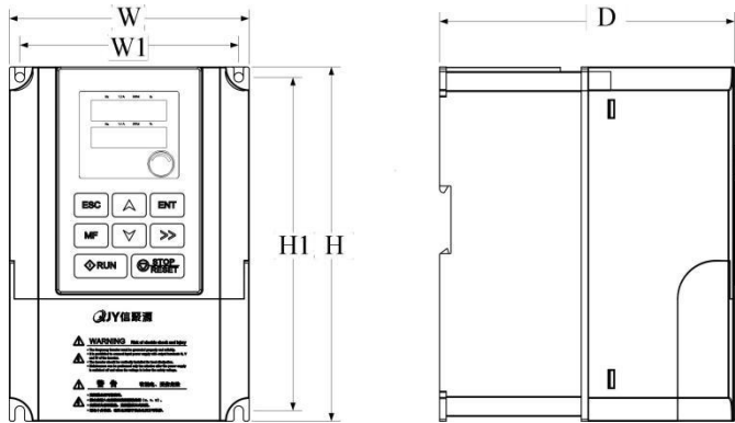
图2-2机箱外形A
