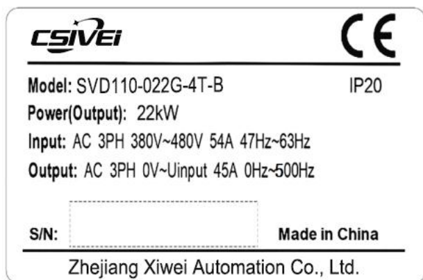
图 2-1 产品铭牌
