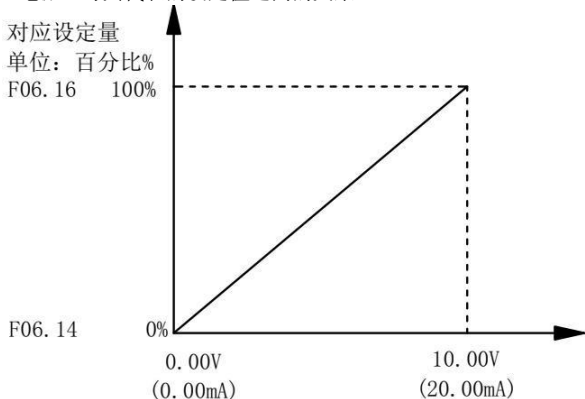
图 6-6 AI1 曲线设定示意图
