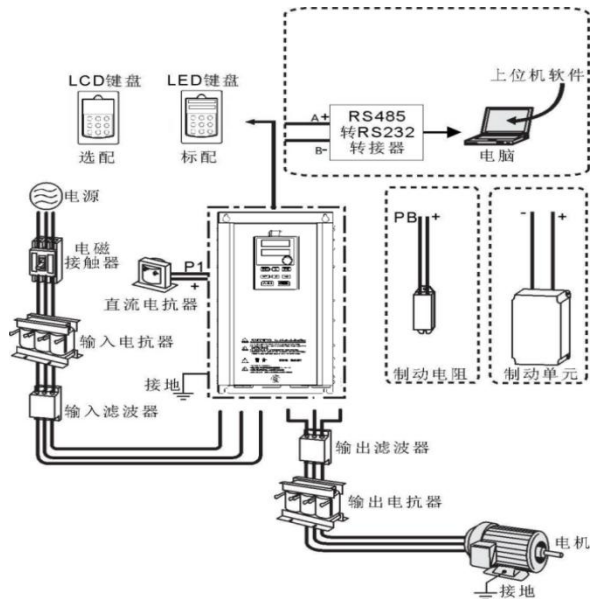
图 3-1 产品外围元器件的标准配置图
