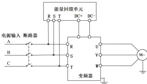
图 3-11 能量回馈单元连接图
