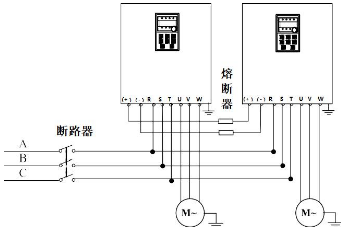
图 3-12 共直流母线的连接
