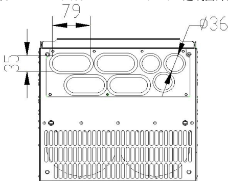
图 3-5 SVD110-132G-4~160G-4 过线圈外形尺寸图 (单位 mm)
