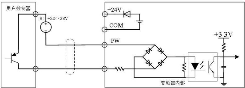
图 3-19 PNP 型拉电流接线方式注：务必去除+24V 与 PW 端子间短路片
