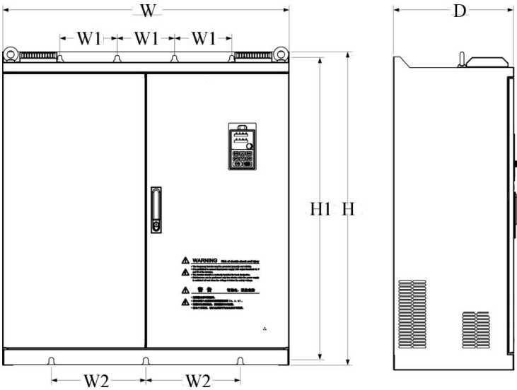
图2-6机箱外形E
