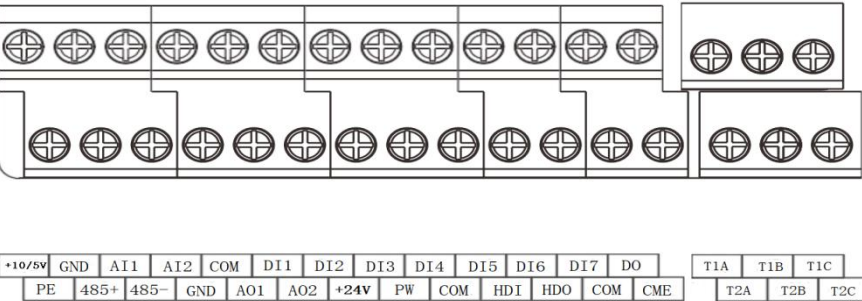
图 3-14 控制板端子示意图
