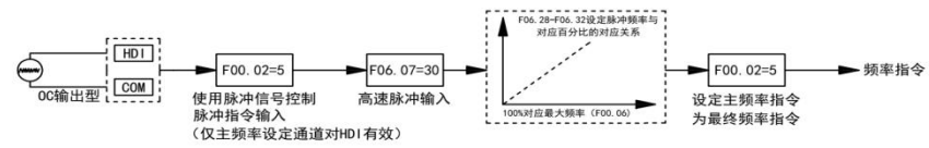
图 6-9 脉冲给定输入主频率参数设置
