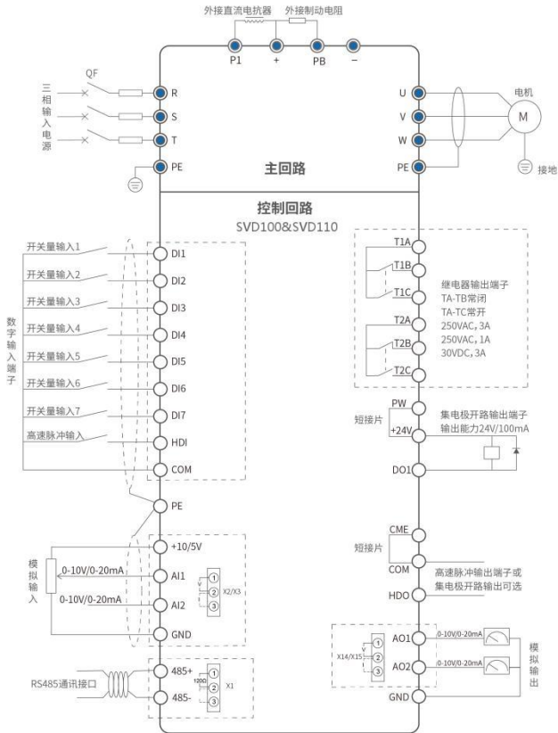
图 3-9 标准接线图
