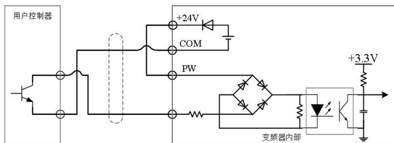
图 3-16 NPN 型灌电流接线方式
