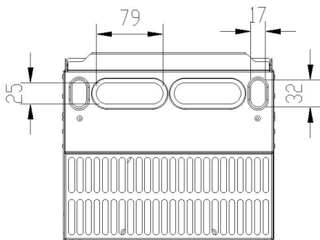
图 3-3 SVD110-37G-4~SVD110-45G-4 过线圈外形尺寸图（单位mm）
