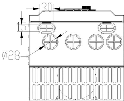
图 3-2 SVD110-18G-4~SVD110-30-4 过线圈外形尺寸图（单位mm）
