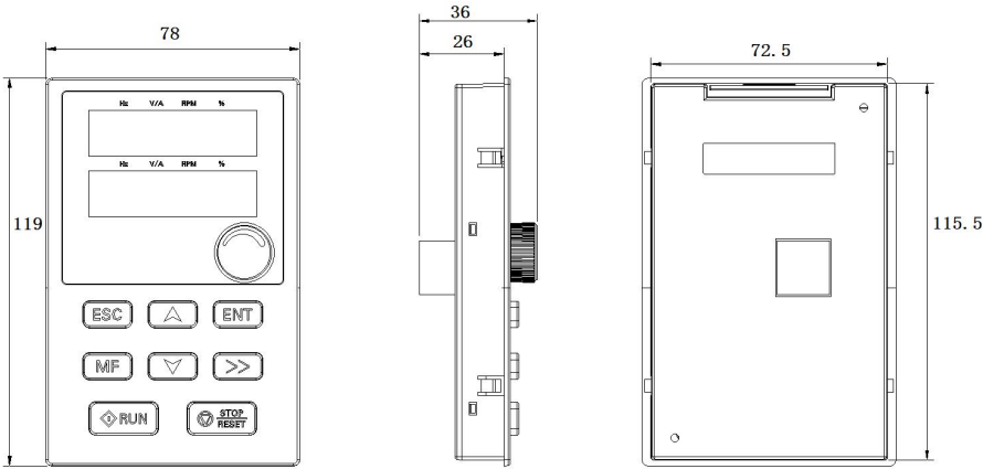
图 2-7 键盘外形及尺寸图（单位mm）
