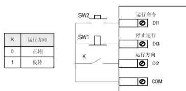
图 6-4 三线式 2
