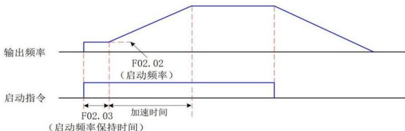
图 6-14 带启动频率的启动时序图
