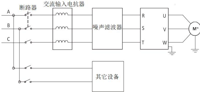
图 3-10 主回路电源侧连接图
