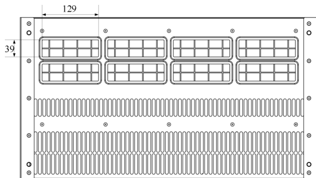
图 3-7 SVD110-315G-4~400G-4 过线圈外形尺寸图（单位 mm）
