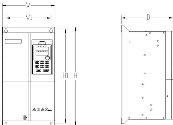
图2-4机箱外形C
