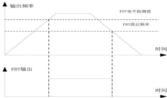
图 6-17 输出频率与FDT 输出关系图
