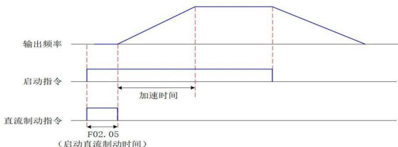
图 6-15 带直流制动的启动时序图
