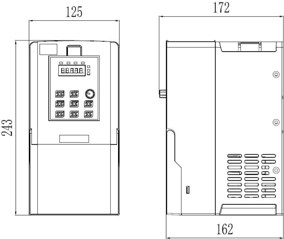
7.5KW 结构示意图及尺寸
