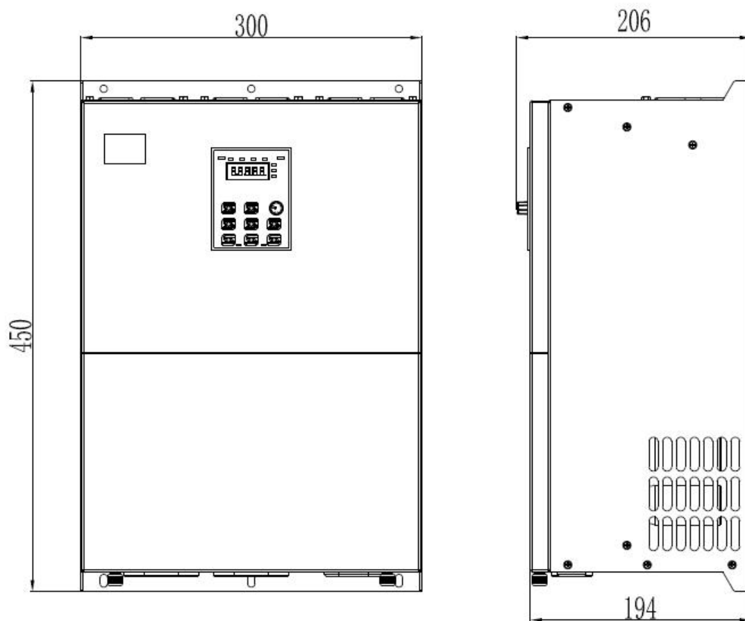
37KW 结构示意图及尺寸
