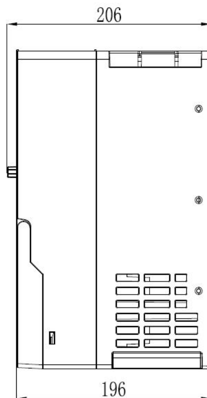
15-22KW 结构示意图及尺寸
