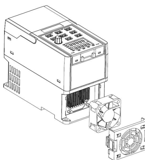
STEP 2 取出风扇并拔出风扇电源端子
