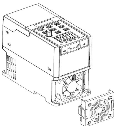
STEP 1 拆卸风扇挡板
