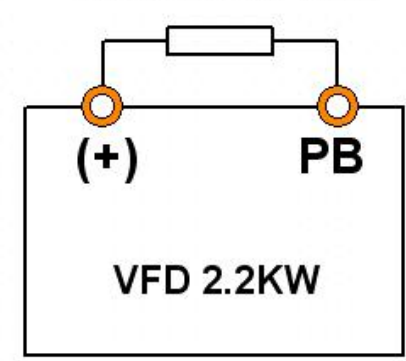
外接制动电阻
