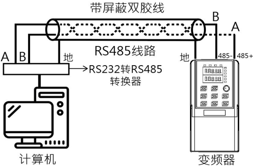
RS485 单机应用时的物理接线图
