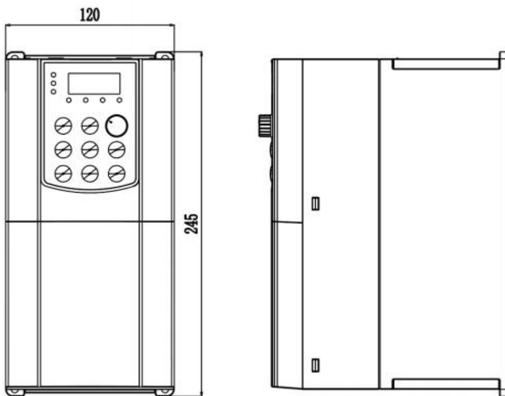
7.5KW 三相单管& 7.5-11KW 三相模组 结构示意图及尺寸
