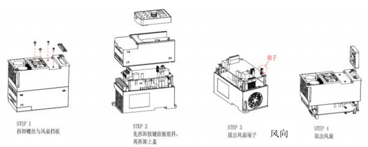
0.75KW~11KW 机器风扇维护示意图
