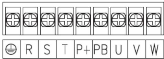
7.5KW 三相主回路端子示意图
