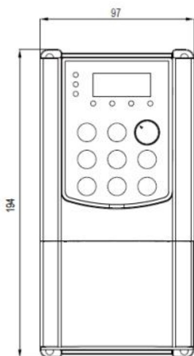
3.7-5.5KW 三相 结构示意图及尺寸
