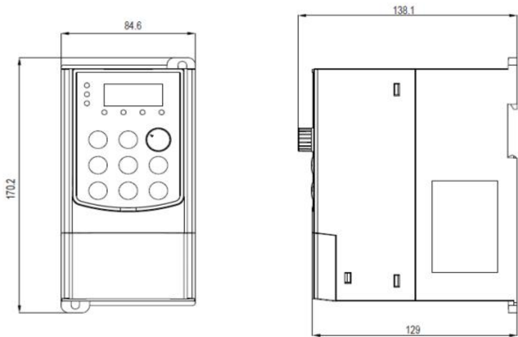
2S 0.75-2.2KW &4T 0.75-2.2KW 结构示意图及尺寸
