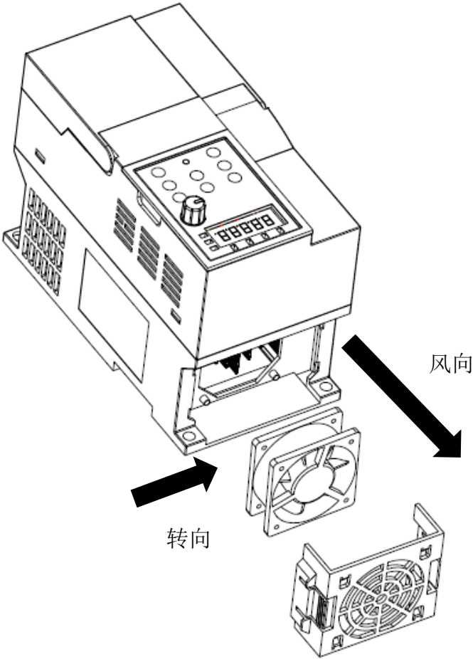
三相 380V 0.75KW~7.5KW 机器风扇维护示意图
