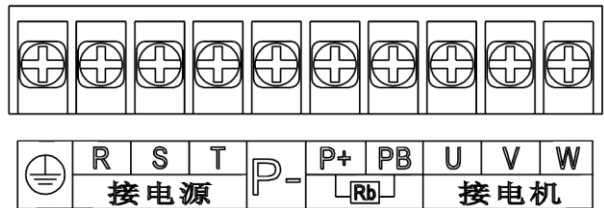
0.75KW-5.5KW 三相主回路端子示意图
