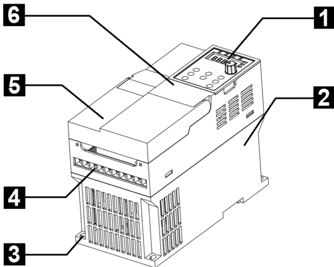
0.75KW—2.2KW 结构示意图及尺寸
