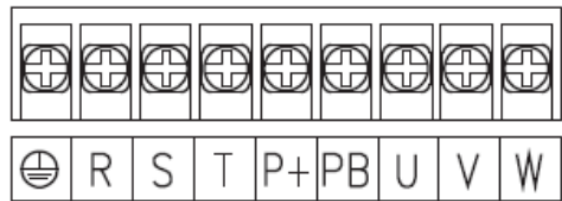
7.5KW 三相主回路端子示意图
