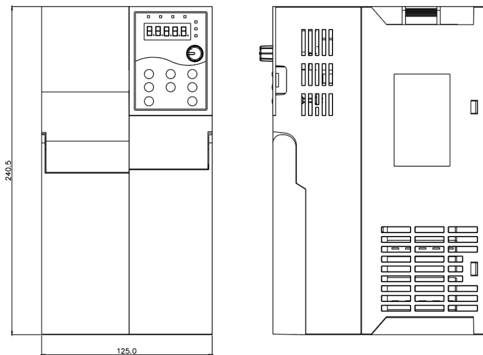
7.5KW 结构示意图及尺寸
