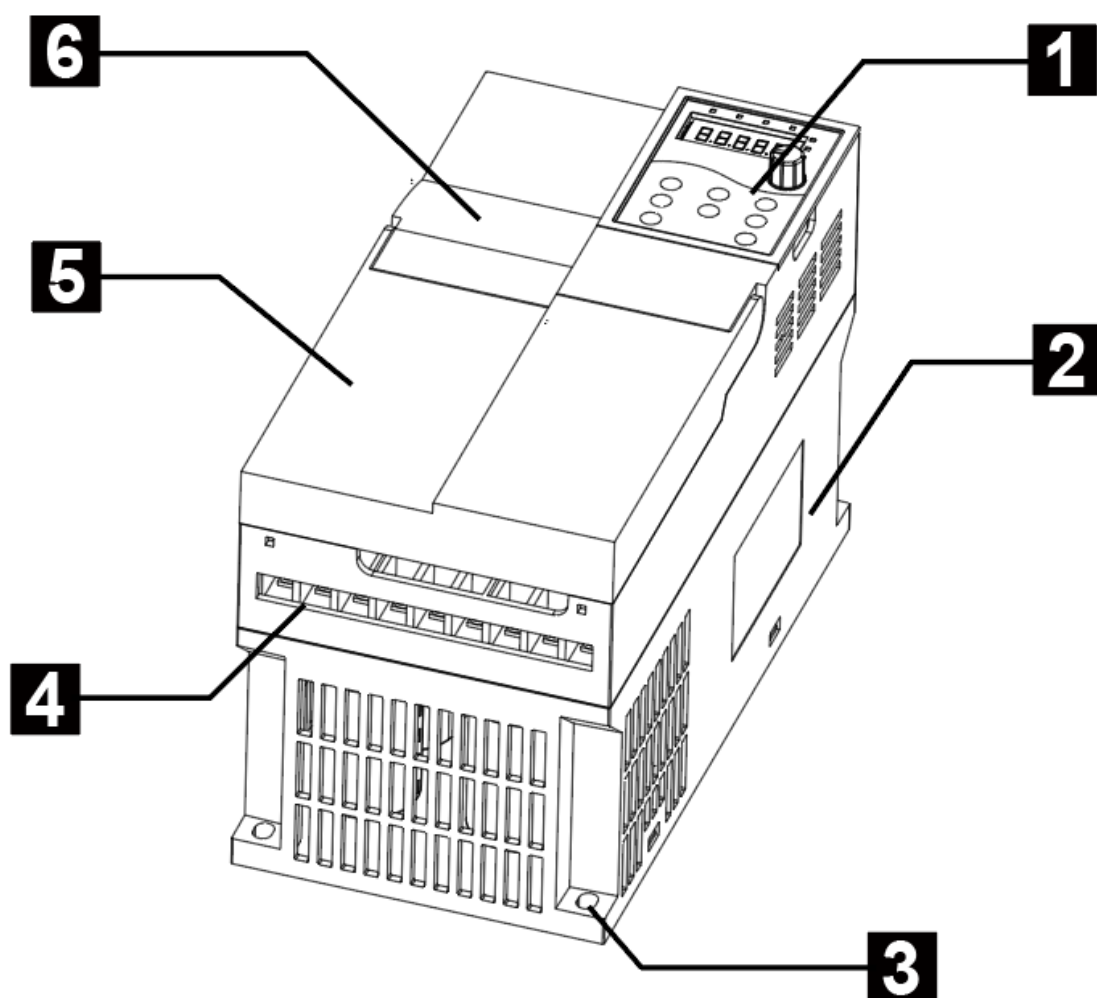
3.7KW—5.5KW 结构示意图及尺寸
